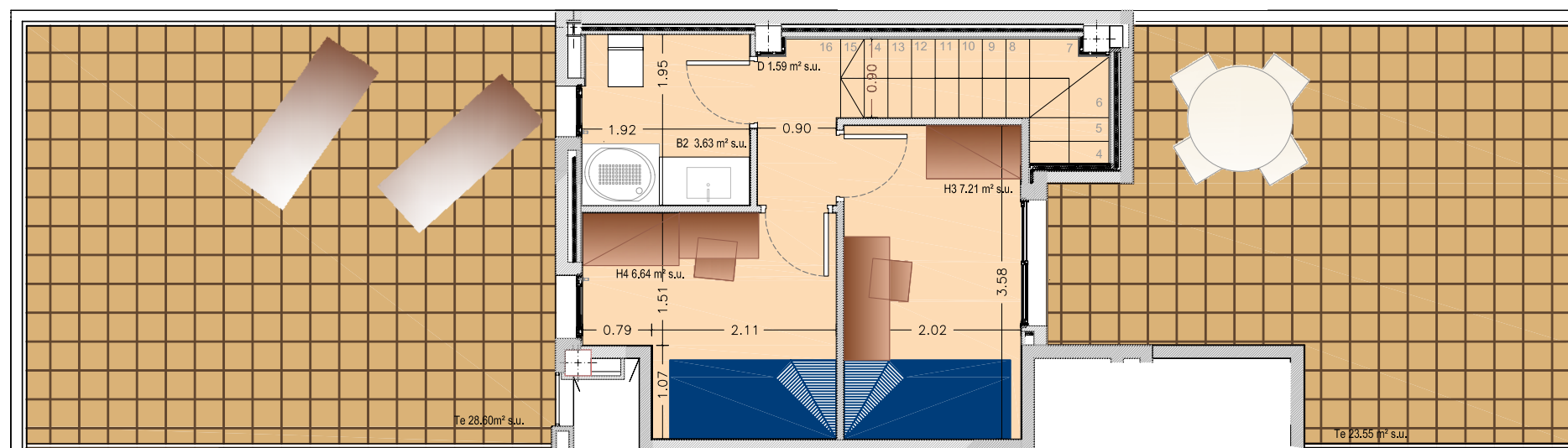
PLANTA SOTACOBERTA
